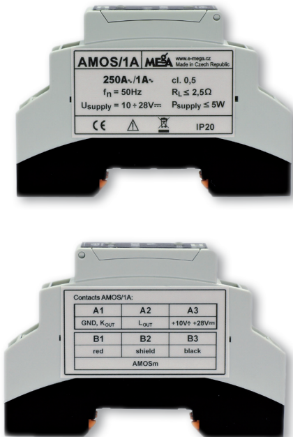
Obr. 1: Informační štítek a štítek se zapojením kontaktů jednotky převodníku AMOS/1A
