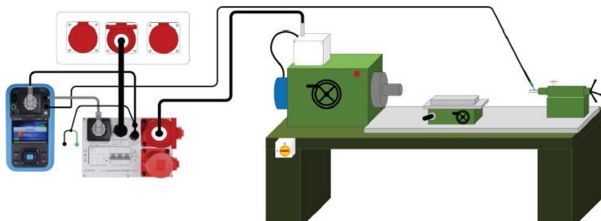
Meranie spojitosti
